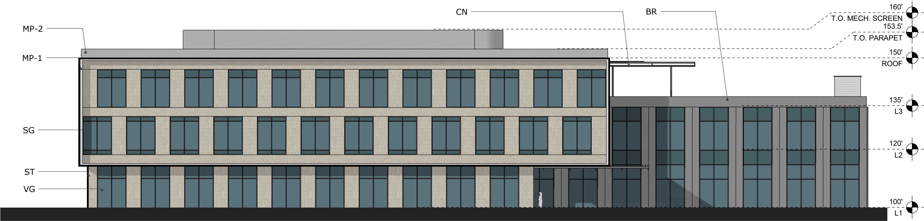
02 East Elevation Scale: 1" : 20'
