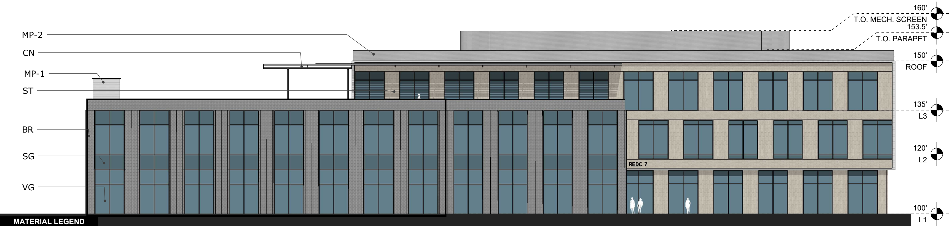
01 West Elevation Scale: 1" : 20'
